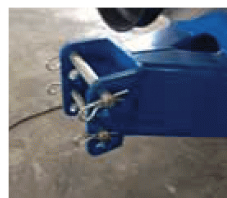
Occhio smontabile e regolabile Removable and adjustable tow-eye Tête d'attelage réglable et amovible
